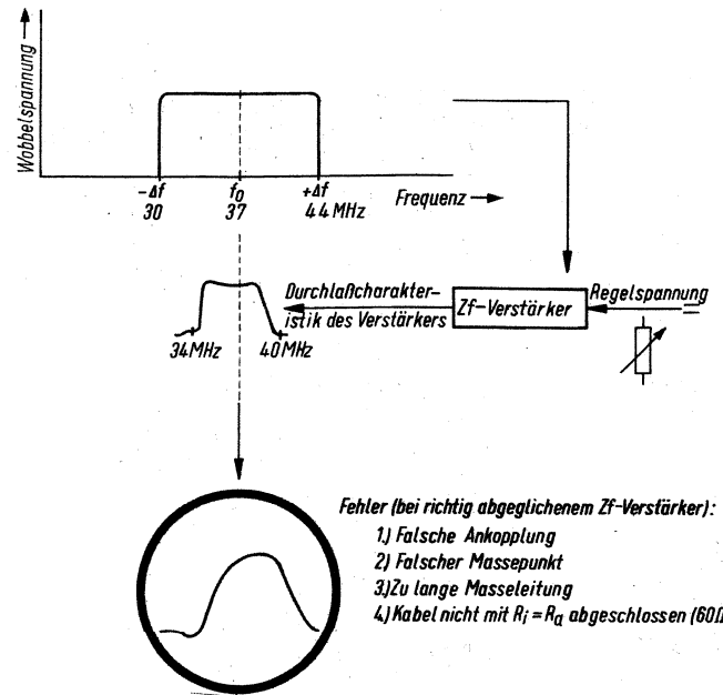
Bild 55. Falsche Durchlaufkurve durch Fehlanpassung des Wobblers
