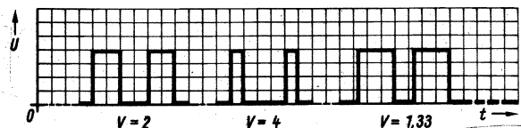
Bild 2.5. Rechteckpulse gleicher Periodendauer mit verschiedenem Tastverhältnis
