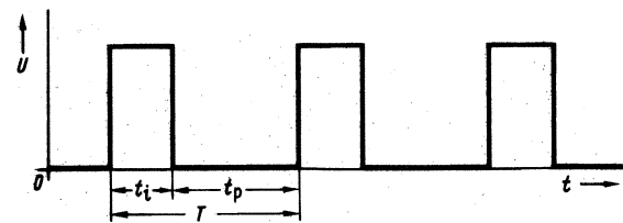
Bild 2.4. Rechteckimpulsfolge oder Rechteckpuls
