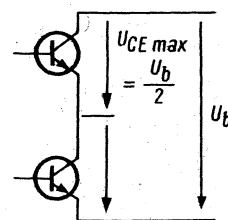
Rechts: Bild 4. Verhältnis von Speisespannung zur zulässigen Kollektoremitter-Spannung in einer übertragerlosen Endstufe
