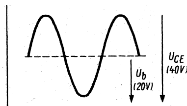
Rechts: Bild 3. Verhältnis von Speisespannung zur zulässigen Kollektoremitter-Spannung in einer Gegentakt-Endstufe
