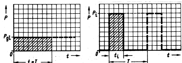
Bild 2.6. Gleichspannung und Pulsperiode gleicher Wirkung
