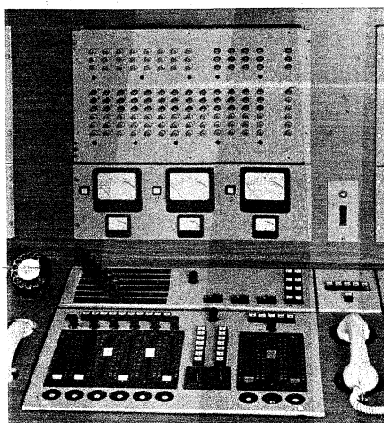
Teilaufnahme des Tisches für die internationale Regie (Intervision, Eurovision) mit Toneinstellern, Aussteuerungskontrolle und Vierdraht-Vermittlung für Fernsprechen (Aufn.: W. Franz KG, Lahr)
