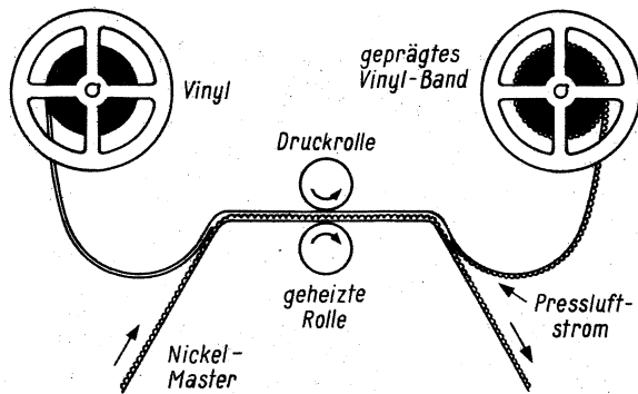
Links: Bild 7. Wie der Nickel-Master das Vinyl-Band prägt
