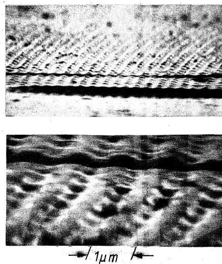
Bild 5. Elektronenmikroskopische Aufnahme der Oberflächenstruktur einer holografischen Selectavision-Aufzeichnung
