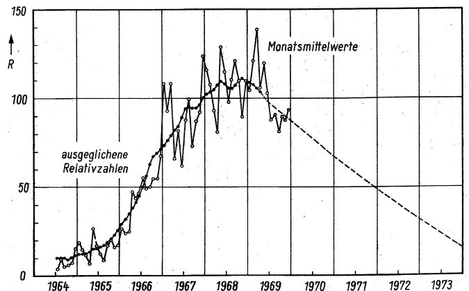
Bild 2. Sonnenfleckenzyklus Nr. 20
