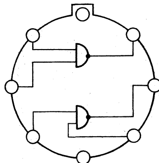
Bild 1a. Der Baustein RTL 914 von SGS mit der in der logischen Schaltungstechnik üblichen Darstellungsart
