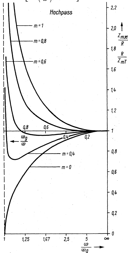
Bild 9. Verlauf von \frac{Z_{m\pi}}{R} und \frac{Z_{mT}}{R} über \frac{\omega_g}{\omega} für verschiedene Werte von m.
