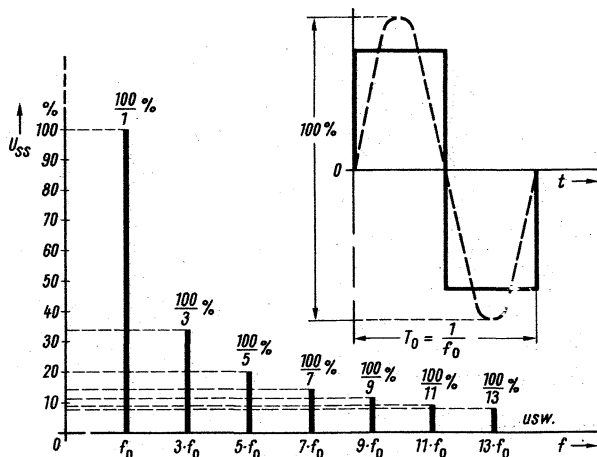
Bild 2.8. Frequenzen und Amplituden der Oberwellen einer Rechteckimpulsfolge
